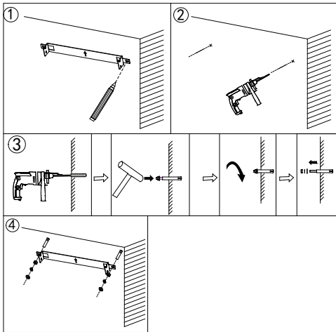
Montagem na parede
