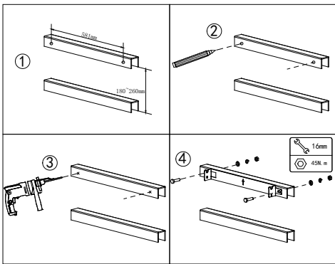
Montagem do suporte
